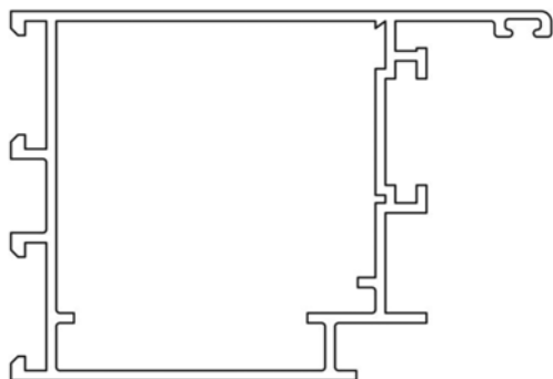
PARANTE PUERTA
