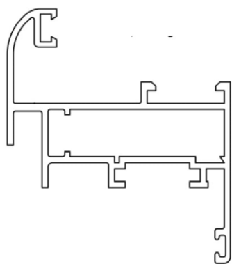
HOJA CURVA DOBLE CONTACTO
