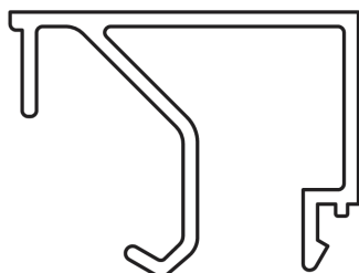
CONTRAVIDRIO RECTO 29MM
